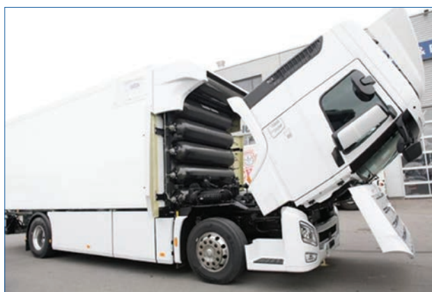
Figure 2 : Camion Hyundai fonctionnant à l'hydrogène – Source : Hyundai.
