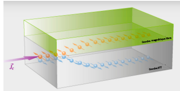
Figure 7 : Schématisation de l'effet Hall de spin.
