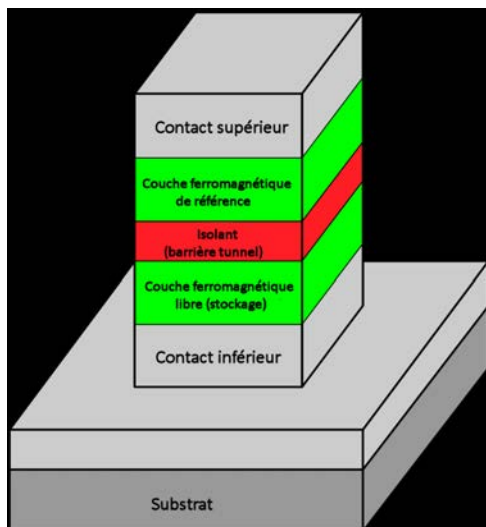
Figure 6 : Schéma d'une jonction tunnel MTJ. Les magnétisations de chacune des couches ferromagnétiques peuvent être orientées par des champs magnétiques externes (créés, par exemple, par des lignes conductrices situées au-dessus et en dessous de la cellule MTJ). Selon que les directions sont parallèles ou anti-parallèles, la cellule laisse ou ne laisse pas passer le courant, ce qui permet de lire ou d'écrire l'information stockée dans la couche libre – Source : d'après Wikipédia.
