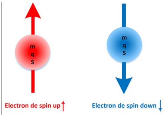
Figure 4 : Le spin des électrons.
