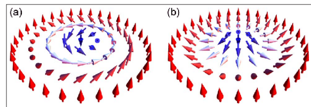
Figure 8 : Schémas de skyrmions de type Bloch (a) et de Néel (b) – Source : Skyrmion-Electronics: An Overview and Outlook. WANG Gang et al., IEEE, octobre, 2016.
